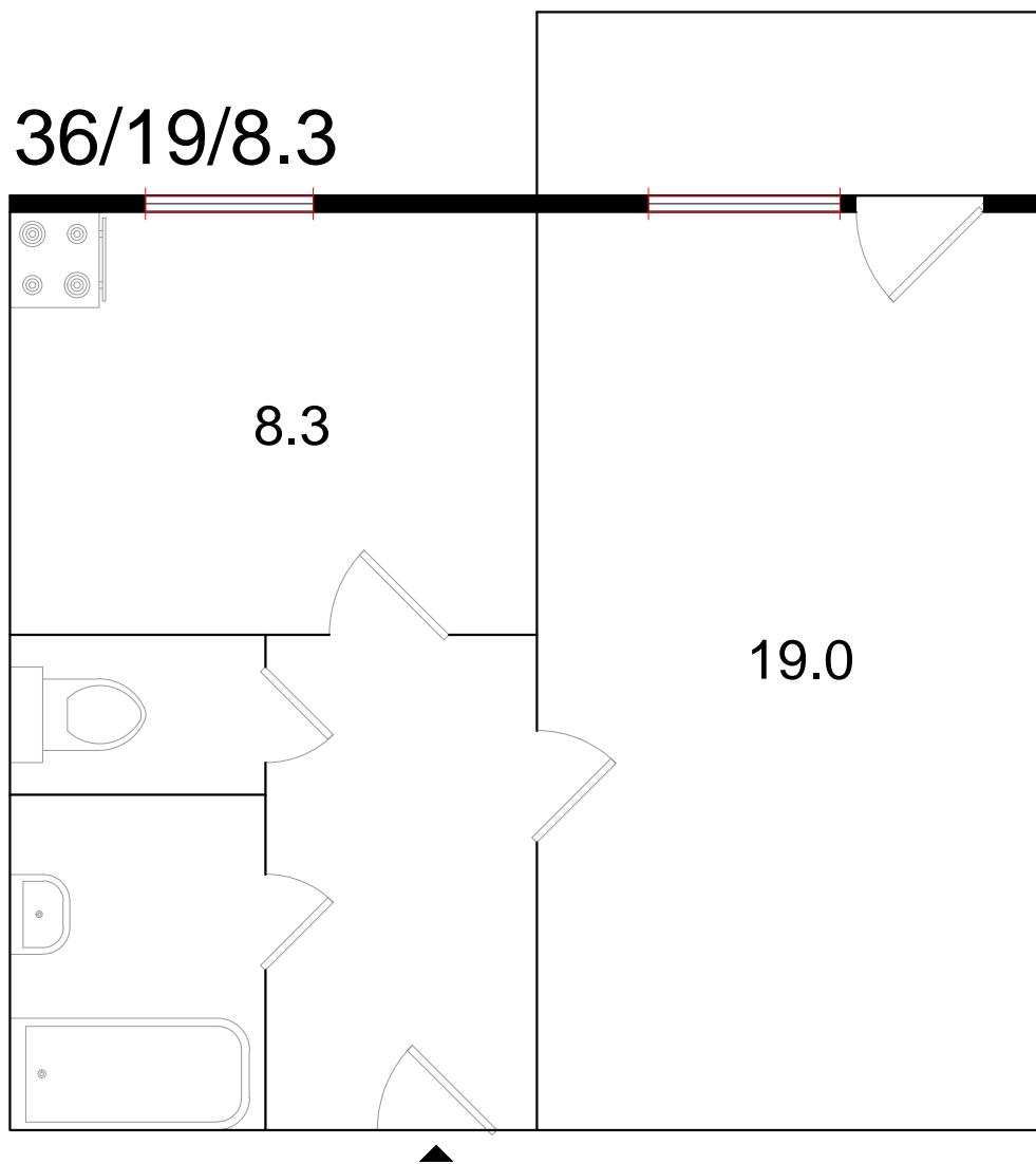
▲ Планировки сталинок. 1-комнатная сталинка (тип 2, серия 1-433)
