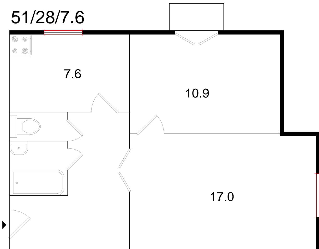
Планировки сталинок. 2-комнатная сталинка (тип 2, серия 1-411)
