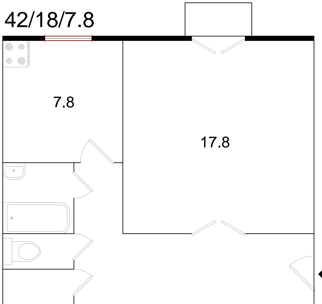
Планировки сталинок. 1-комнатная сталинка (тип 1, серия 1-411)
